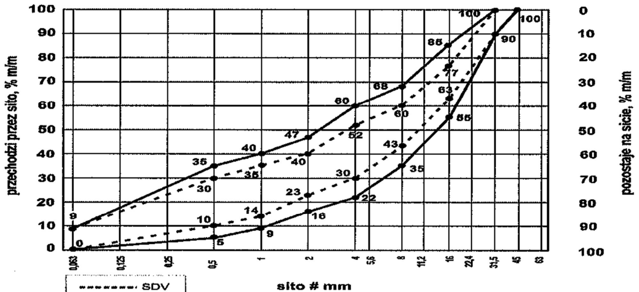
Rys. 12. Mieszanka niezwiązana 0/31, 5 do warstw podbudowy zasadniczej
