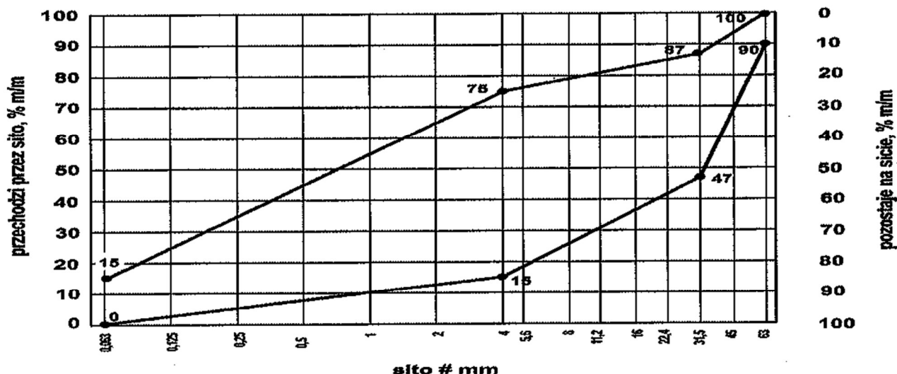
Rys. 8. Mieszanka kruszyw 0/63
