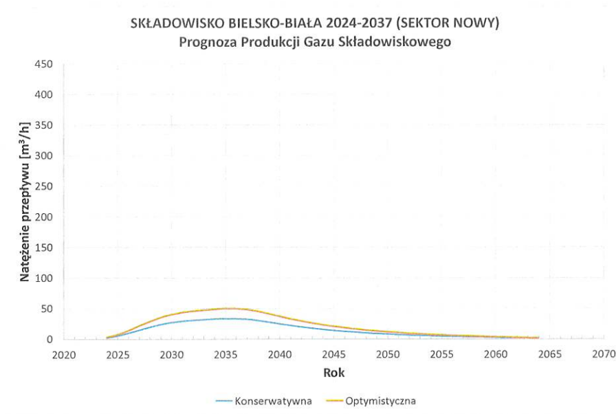
Rysunek 1 Wykres prognozy produkcji biogazu składowiskowego – sektor nowy
